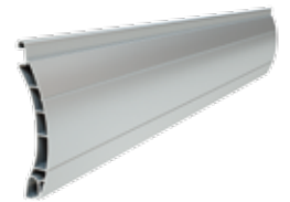
PT 52 | wysokość profilu: 52 mm grubość: 14 mm
